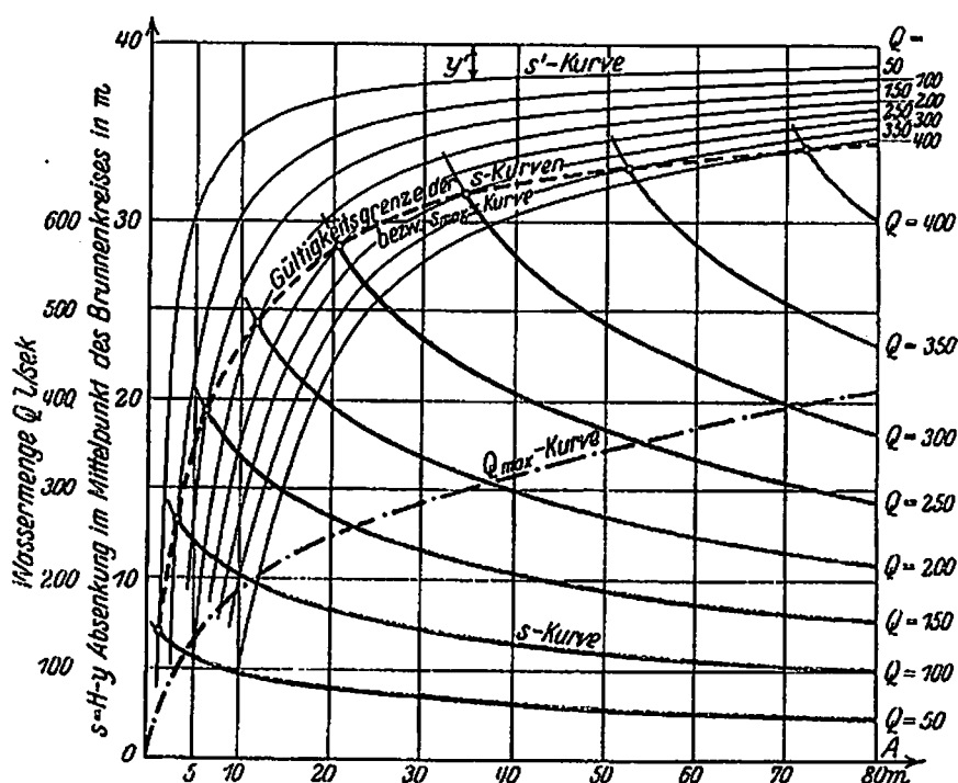
Abb. 39. Absenkung über einer undurchlässigen Schicht. Größtwerte der zu erreichenden Absenkung s_{\max} und des zu bewältigenden Wasserandranges in Abhängigkeit vom Brunnenkreishalbmesser A .
