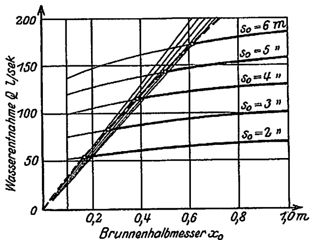
Abb. 20. Wasserentnahme Q in Abhängigkeit vom Brunnenhalbmesser x_0 bei konstanter Absenkung s_0 im Brunnen nach Kyrioleis, jedoch unter Berücksichtigung des Brunnenfassungsvermögens.
