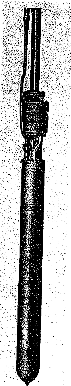
Abb. 6. Motorsenkpumpe für Tiefbrunnen. Die bei der Grundwasserabsenkung für den Umbau und die Erweiterung der Staatsoper Unter den Linden in Berlin zur Verwendung gekommene Tauchmotorpumpe der Siemens-Schuckertwerke.
