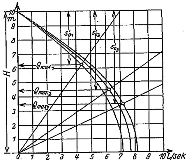
Abb. 17. Einfluß der Änderung des Brunnenhalbmessers auf die Größe der tiefsten Absenkung.
