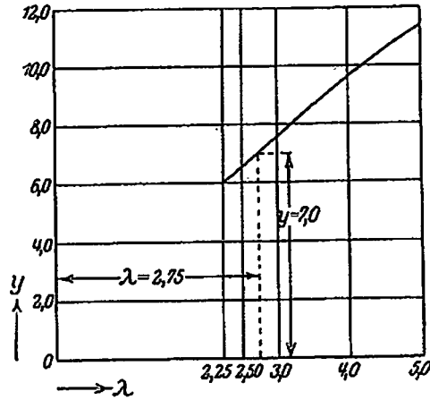
Abb. 40. Graphische Bestimmung des Wertes \lambda bzw. des Brunnenabstandes ( b = \lambda \cdot 2x_0 ) für den Fall, daß die Größen A , s und y festliegen.
