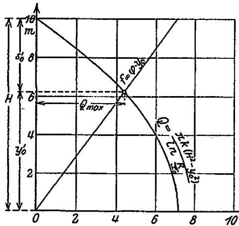
Abb. 16. Graphische Ermittlung des tiefsten Absenkungszustandes für den Einzelbrunnen.
