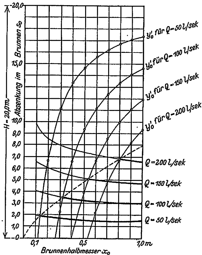
Abb. 18. Absenkung s_0 in einem Brunnen in Abhängigkeit vom Brunnenhalbmesser x_0 bei konstanter Wasserentnahme Q nach Kyrielleis, jedoch unter Berücksichtigung des Fassungsvermögens.
