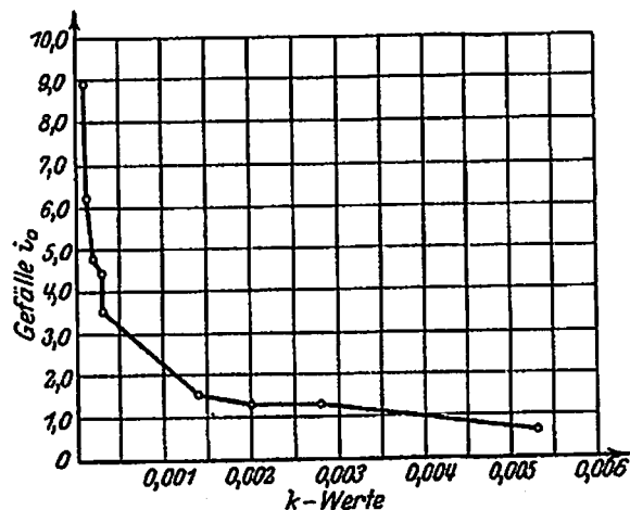
Abb. 14. Beziehungen zwischen dem Grenzgefälle i_0 am Brunnen und dem k -Wert gemäß Zahlentafel 4.
