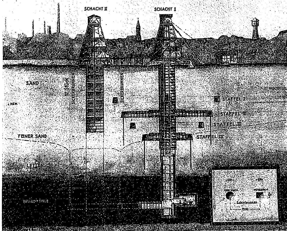
Abb. 5. Grundwasserabsenkung für die Doppelschachtenanlage der Matador-Bergbaugesellschaft m. b. H. bei Senftenberg (Nieder-Lausitz), nach dem Verfahren der Siemens-Bauunion, Berlin. (Entnommen aus Mitteilungen der Siemens-Bauunion 1927.)
