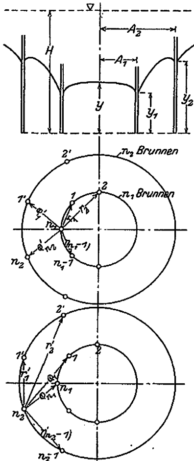
Abb. 24. Mehrbrunnenanlage von kreisförmigem Grundriß mit zwei konzentrischen Brunnenstaffeln in Betrieb.
