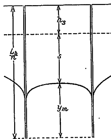
Abb. 38. Bohrtiefe der Brunnen.
