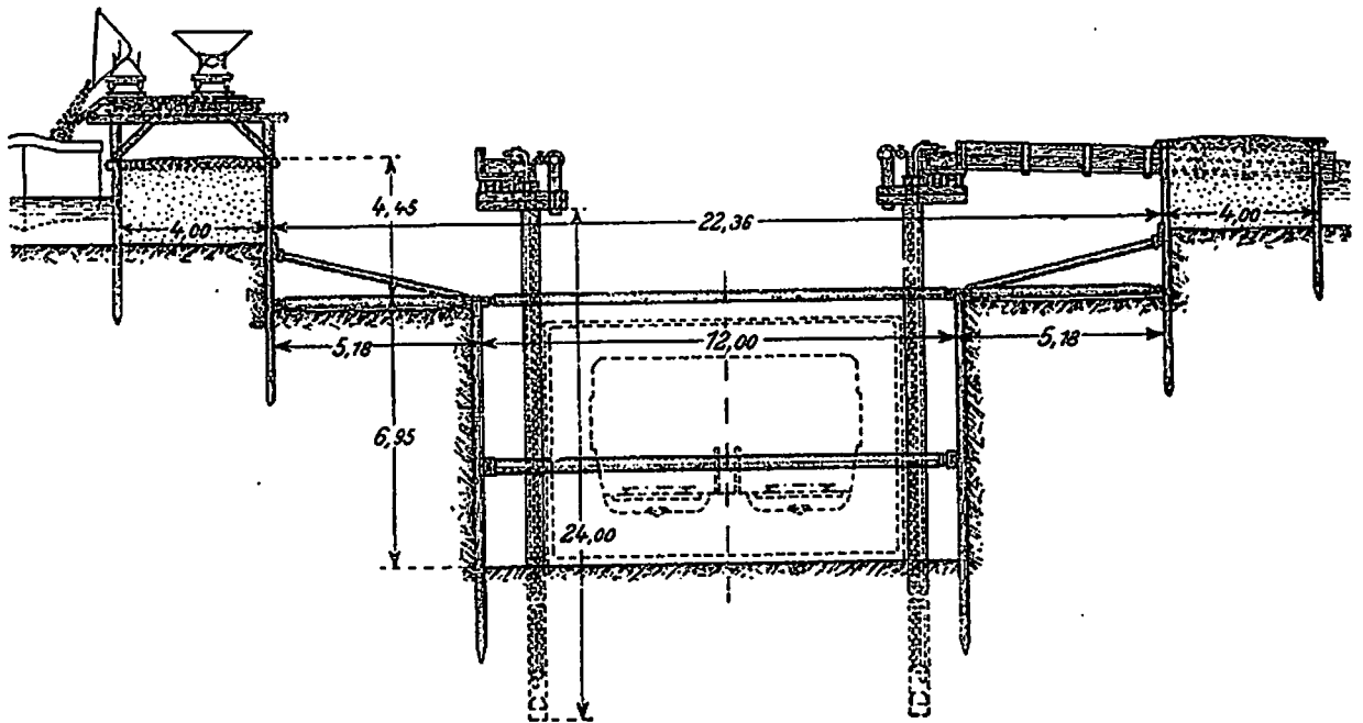
Abb. 2. Mammutpumpenanlage beim Bau des Sprectunnels an der Inselbrücke in Berlin. Querschnitt durch die Baugrube. (Entnommen aus Siemens-Zeitschrift April 1927.)
