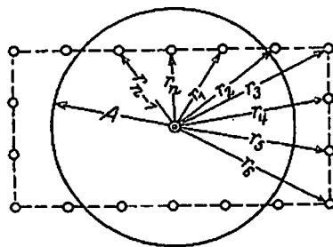
Abb. 21. Ersatz der wirklichen Grundrißanordnung der Brunnen (von beliebiger Gestalt) durch einen gedachten Brunnenkreis (Ersatzkreis).
