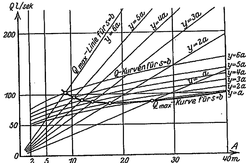
Abb. 36. Konstruktion der Q_{max} -Kurve für verschiedene Eintauchtiefen der Brunnen. Beispiele: s = b ; y = a, 2a, 3a, 4a, 5a, 6a .
