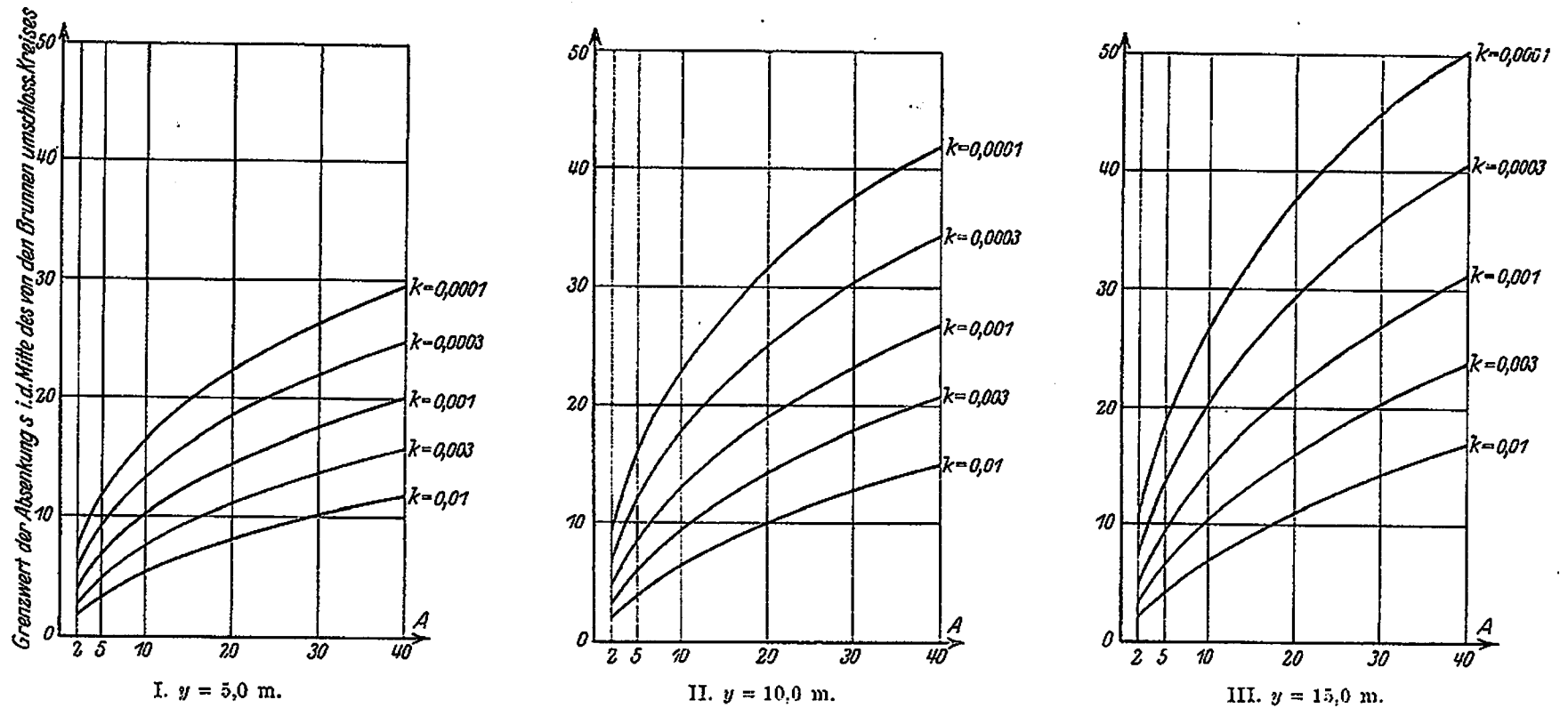
Abb. 34. Tiefste Absenkung s in der Mitte des Brunnenkreises bei voller Ausnutzung des Fassungsvermögens in Abhängigkeit vom Halbmesser A des Brunnenkreises für verschiedene k -Werte; x_0 = 0,1 m; \lambda = 5,00 .
