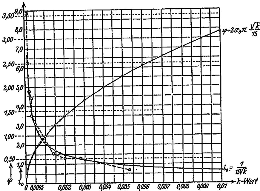
Abb. 15. Beziehungen zwischen dem Grenzgefälle i_0 , dem Passungswert \varphi und dem k -Wert unter Zugrundelegung der Formeln i_0 = \frac{1}{15\sqrt{k}} und \varphi = 2\pi\sqrt{k} \frac{\sqrt{k}}{15} .
