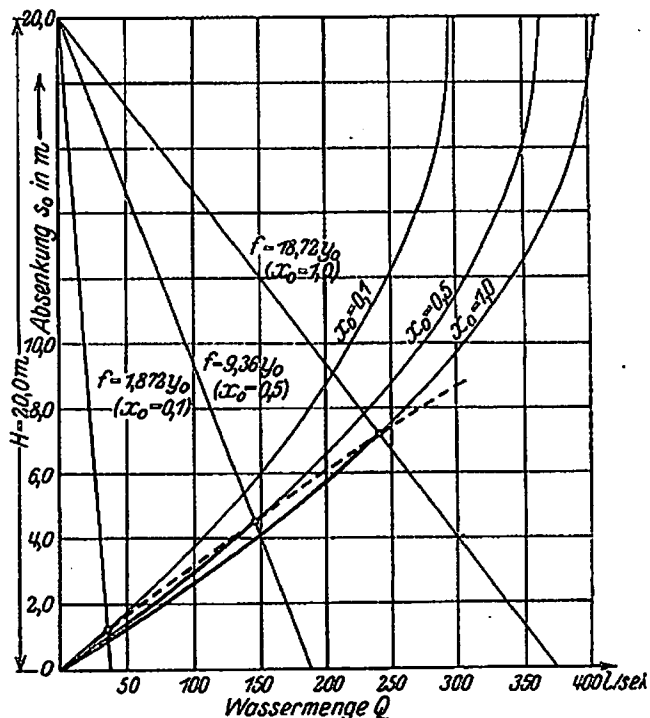
Abb. 19. Absenkung s_0 in einem Brunnen von bestimmtem Halbmesser x_0 in Abhängigkeit von der Wasserentnahme Q nach Kyrioleis, jedoch unter Berücksichtigung des durch das Brunnenfassungsvermögen gegebenen Geltungsbereichs.
