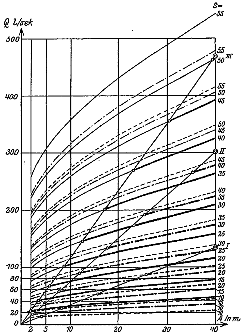
Abb. 35. Abhängigkeit des von der Absenkungsanlage aufzunehmenden Wasserandranges Q von der Absenkungstiefe s , dem Halbmesser des Brunnenkreises und dem Wasserstand y in der Mitte des Brunnenkreises über den Brunnensohlen.
