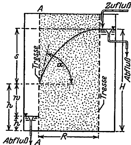
Abb. 13. Versuchsanordnung zur Beobachtung des Grenzgefälles des Grundwasserspiegels.
