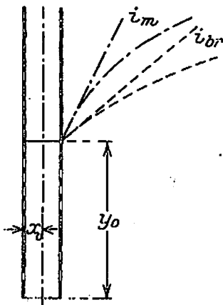
Abb. 9. Spiegelgefälle am Brunnenmantel.
