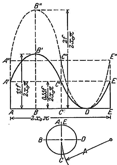
Abb. 33. Drosselung des Fassungsvermögens bei zu geringem Brunnenabstand, dargestellt durch Auftragung der auf den laufenden Zentimeter des abgewickelten Brunnenumfangs entfallenden Sickermenge.
