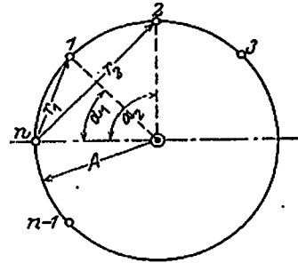
Abb. 23. Beziehungen zwischen den Strahlen r und dem Brunnenhalbmesser A sowie dem Zentriwinkel \alpha .
