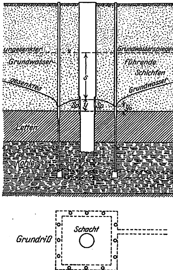
Abb. 11. Sickerbrunnenanlage der Matador-Bergbau-gesellschaft in Senftenberg (Nieder-Lausitz).
