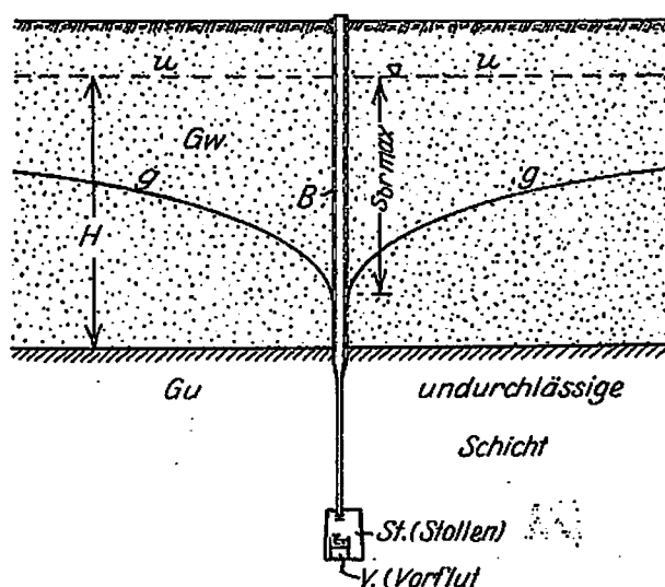
Abb. 10. Anordnung eines Sickerbrunnens.
