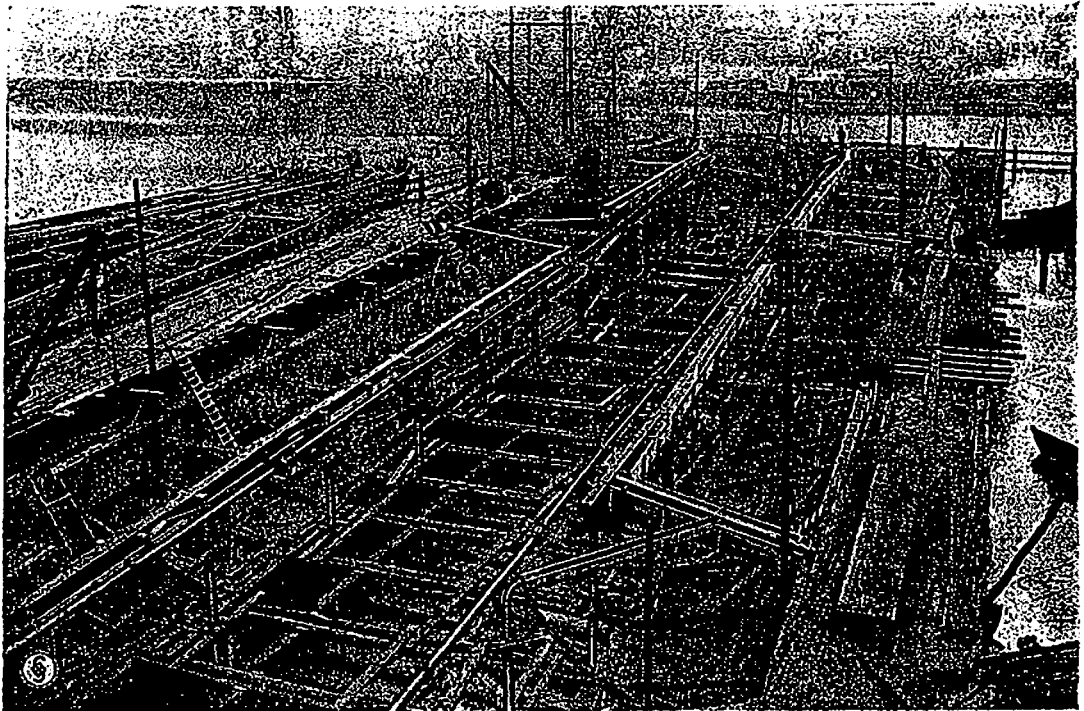
Abb. 1. Mit Mammutpumpen betriebene Tiefbrunnenanlage beim Bau des Sprectunnels an der Inselbrücke in Berlin. (Entnommen aus Siemens-Zeitschrift April 1927.)
