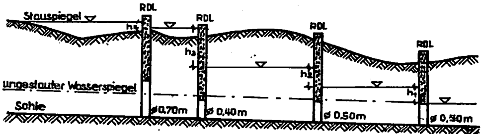
Abb. 4 Aufstau durch mehrere zum Teil falsch dimensionierte Rohrdurchlässe (Addition der Stauwerte h_1 + h_2 + h_3 + h_4 ) RDL = Rohrdurchlaß
