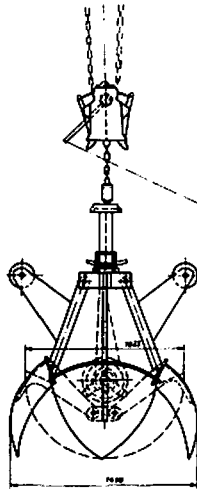
Vierschalengreifer Taatz
