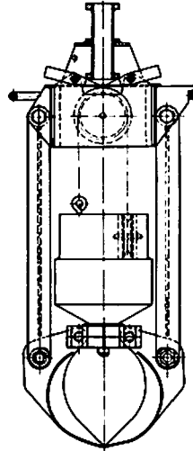
Sechschalengreifer
