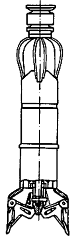
Benotgreifer
