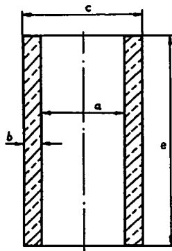
Splittbetonfilter ohne Fals
