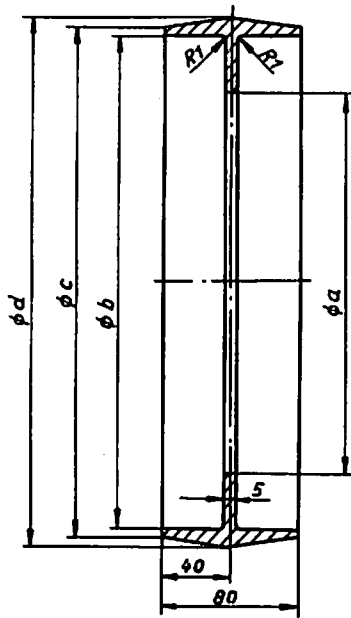
Abmessungen (mm)
