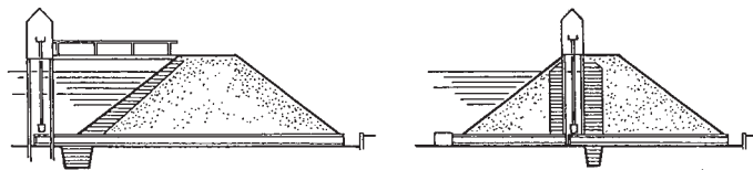
Die Lage der Rasenhauptdichtung und die Stellung des Striegelhäuschens bei der ursprünglichen und bei der neuen Dammbauweise.
